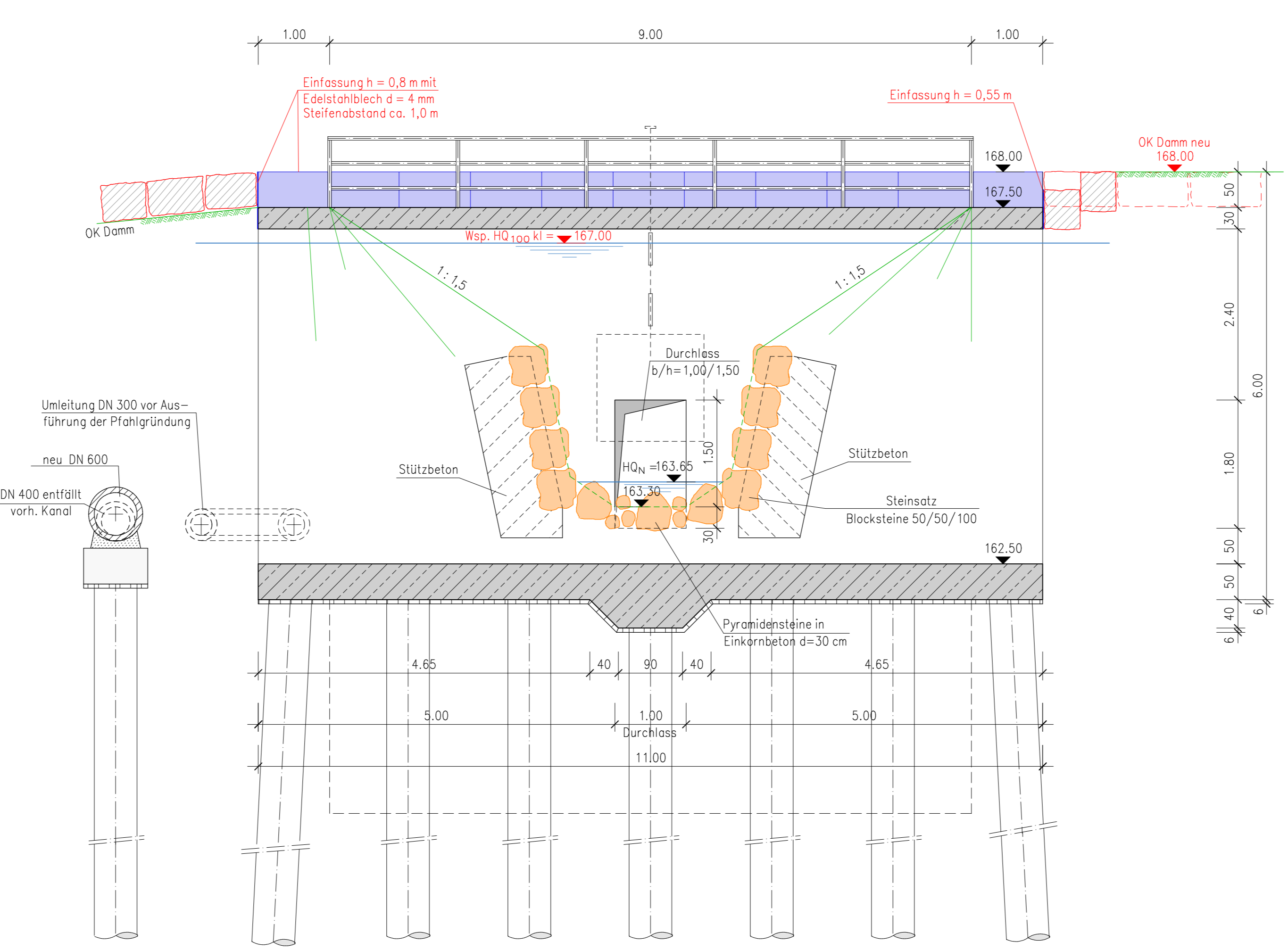
Schnitt 3 - 3 M. 1 : 50
