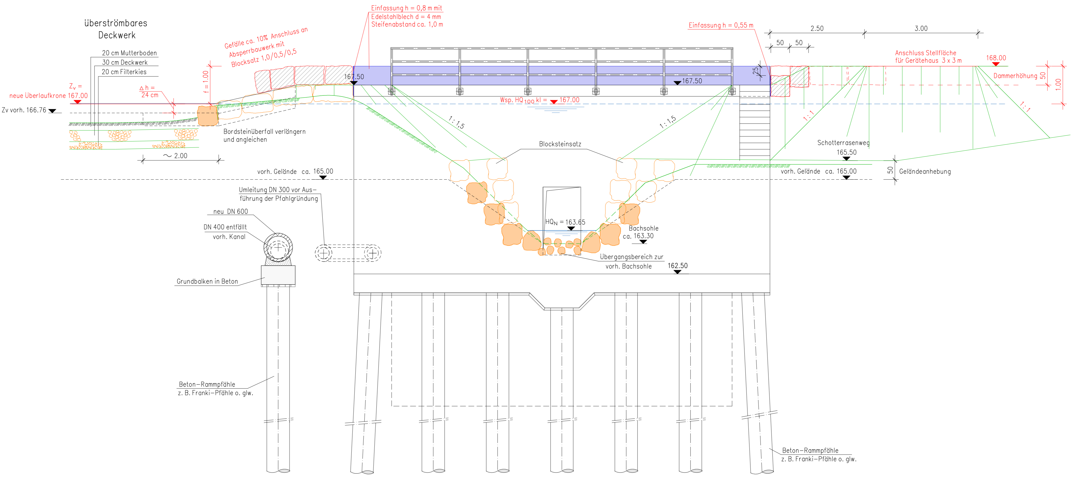
Schnitt 5 - 5 M. 1 : 50
