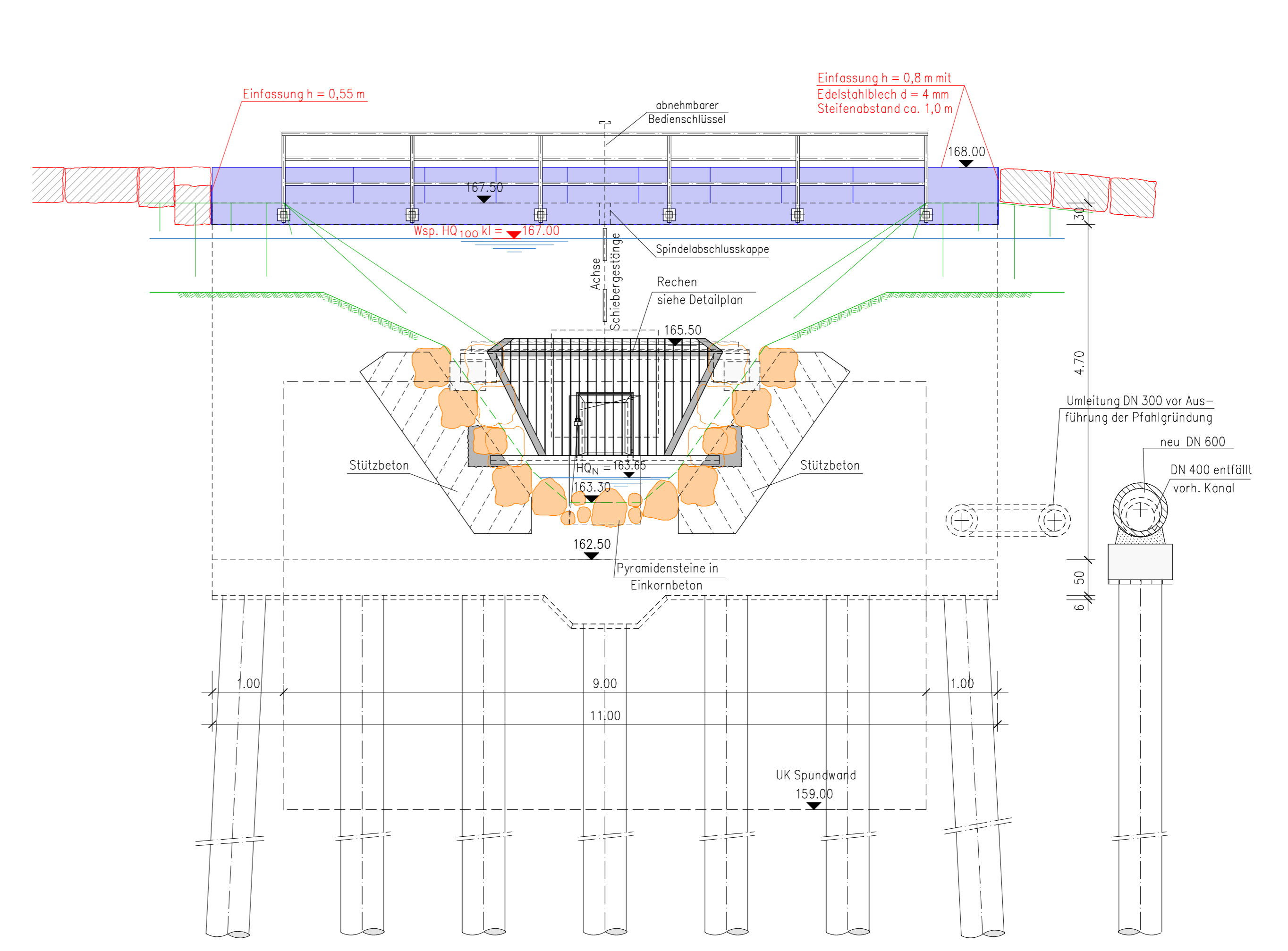
Schnitt 4 - 4 M. 1 : 50
