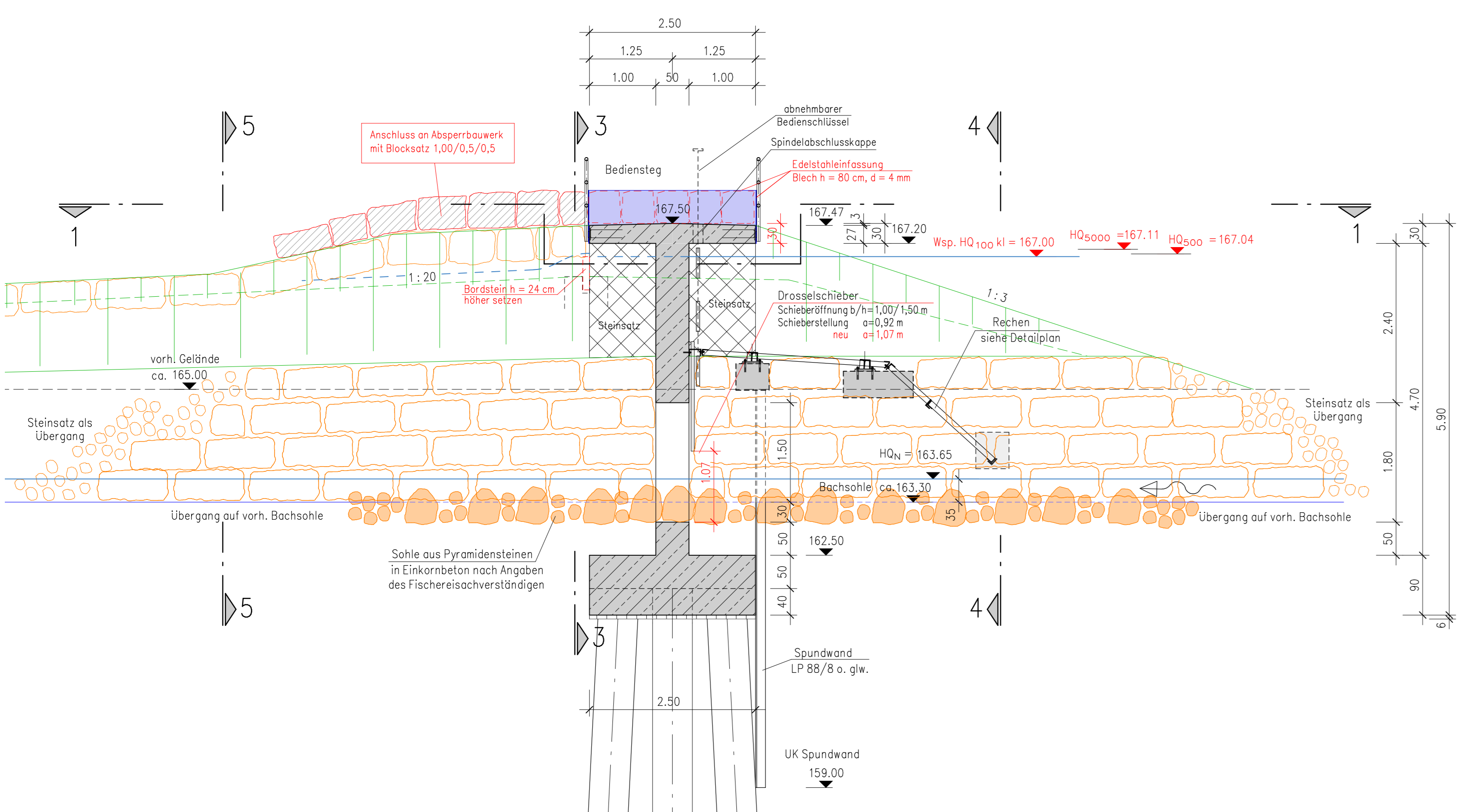
Schnitt 2 - 2 M. 1 : 50 (überströmbarer Damm 1)
