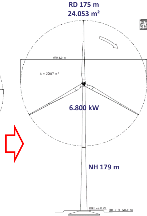
WEA VI 267 m Gesamthöhe ca. > 16 Mio. kWh/a
