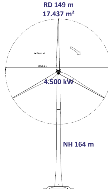
Bretzfeld-Obersulm 239 m Gesamthöhe ca. 12 Mio. kWh/a
