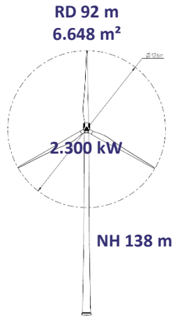
Windpark Löwenstein 184 m Gesamthöhe ca. 6 Mio. kWh/a
