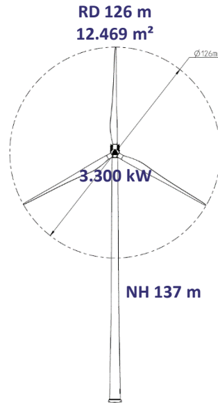
Windpark Weißbach 200 m Gesamthöhe ca. 7 Mio. kWh/a
