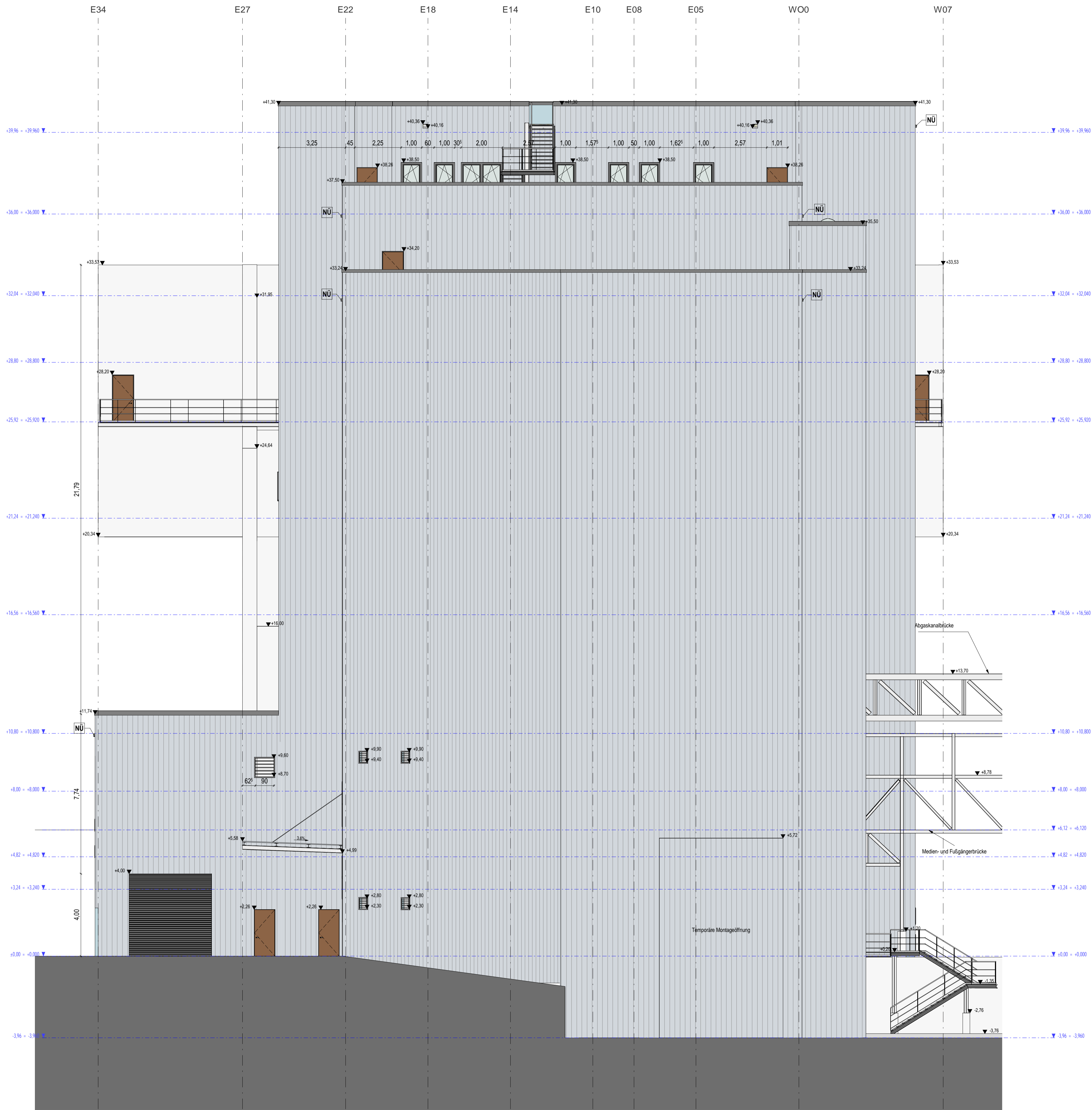
Ansicht Nord
