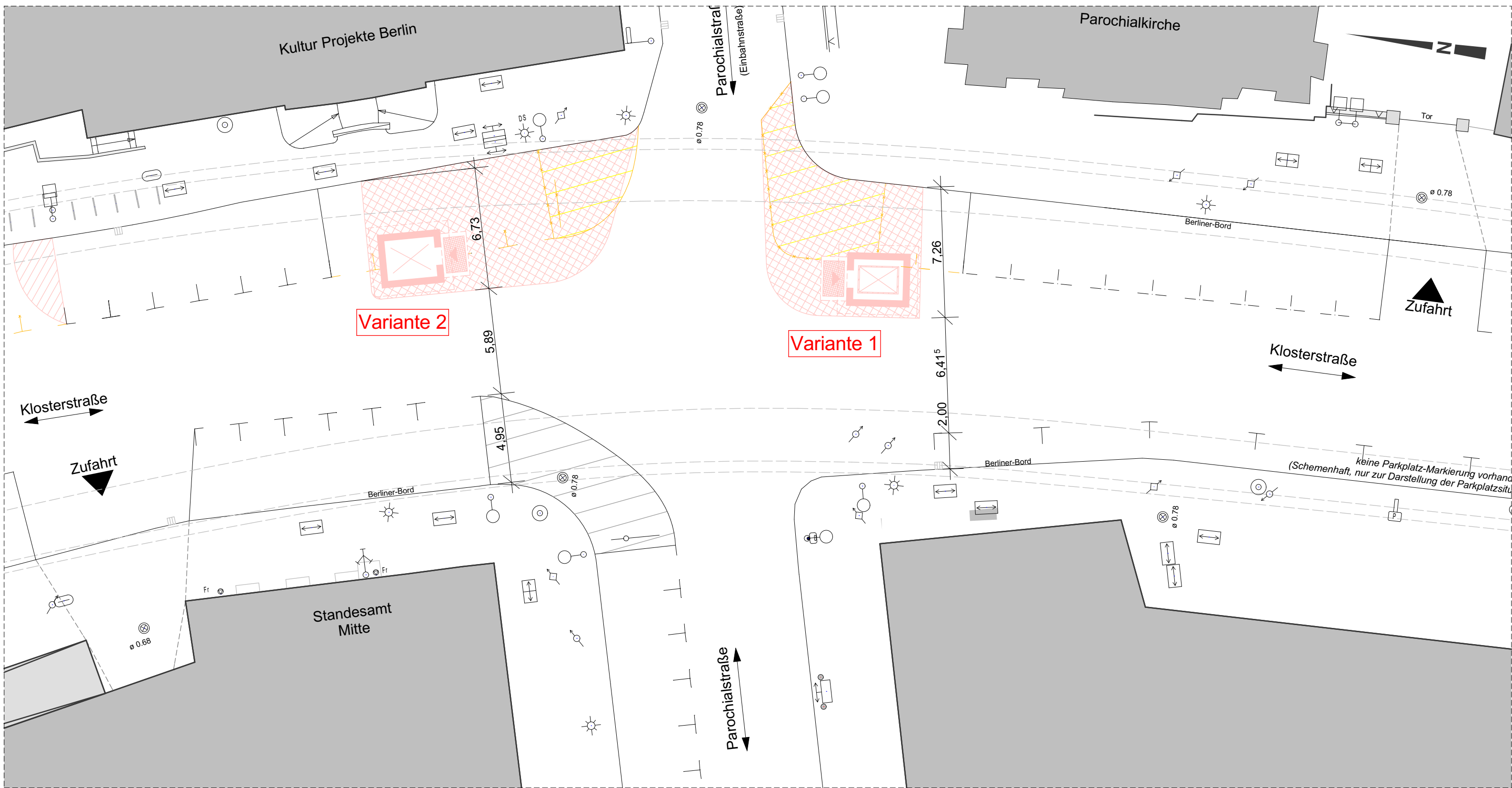
Lageplan Auszug, Aufzugsvarianten 1 und 2, M 1:200
