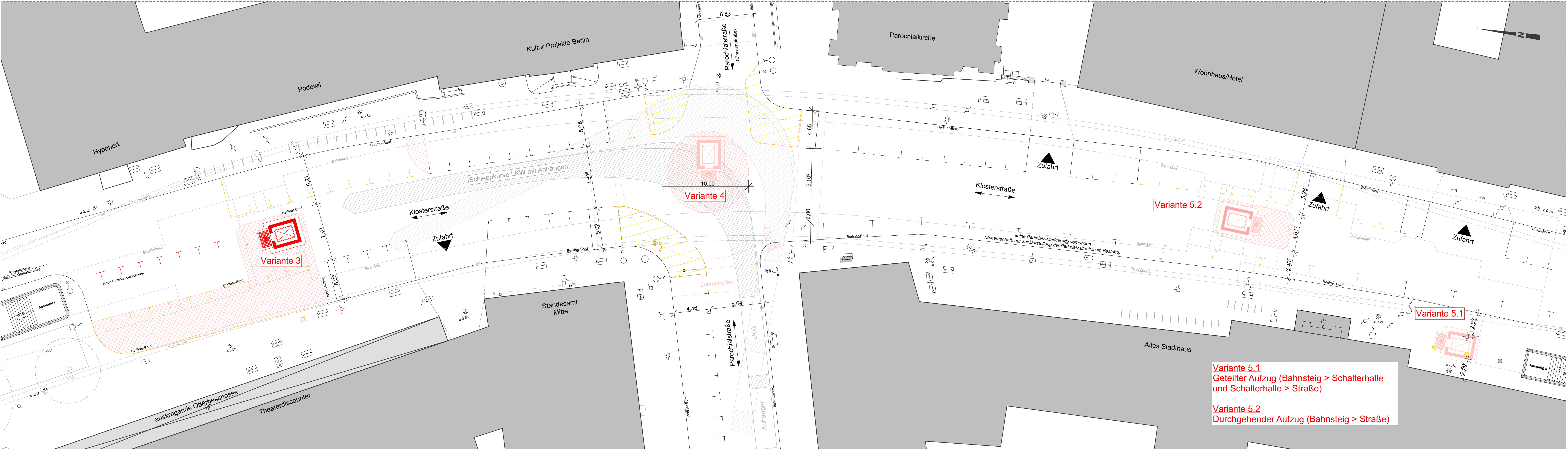
Lageplan, Aufzugsvarianten 3,4,5.1 und 5.2, M 1:200
