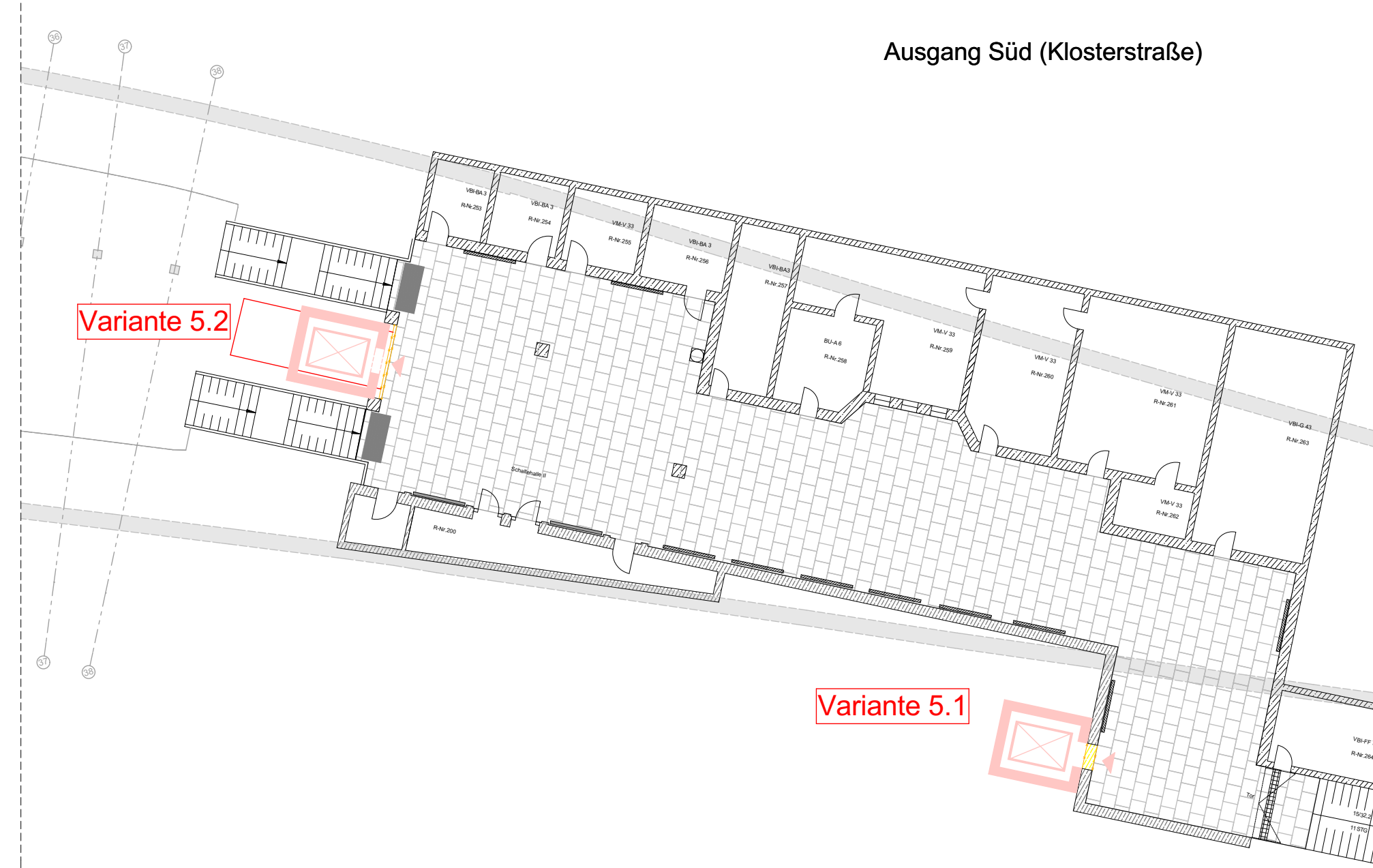
Schalterhallen II, Aufzugsvarianten, M 1:200
