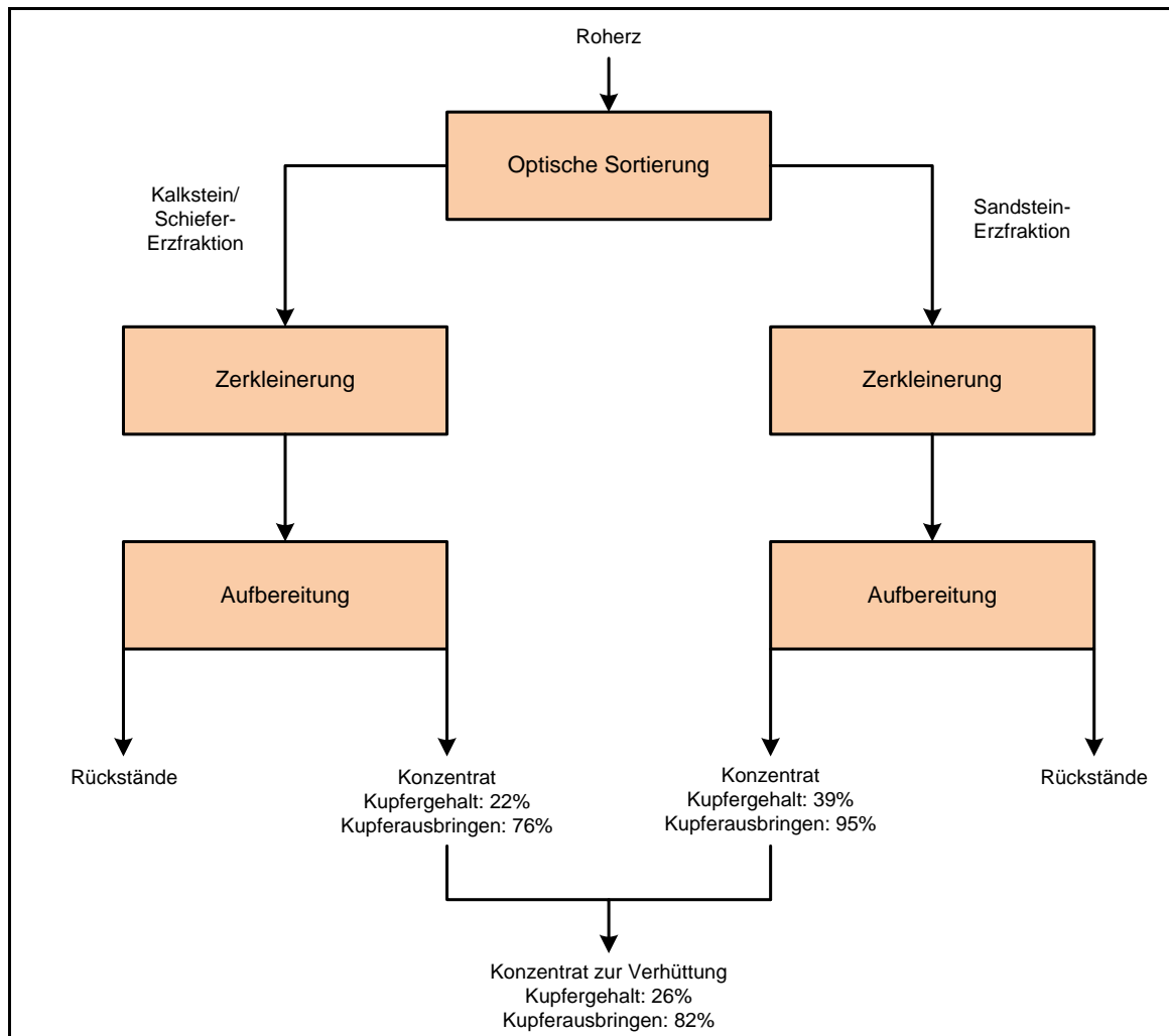
Abbildung 4: Grundfließbild zum Aufbereitungsprozess
