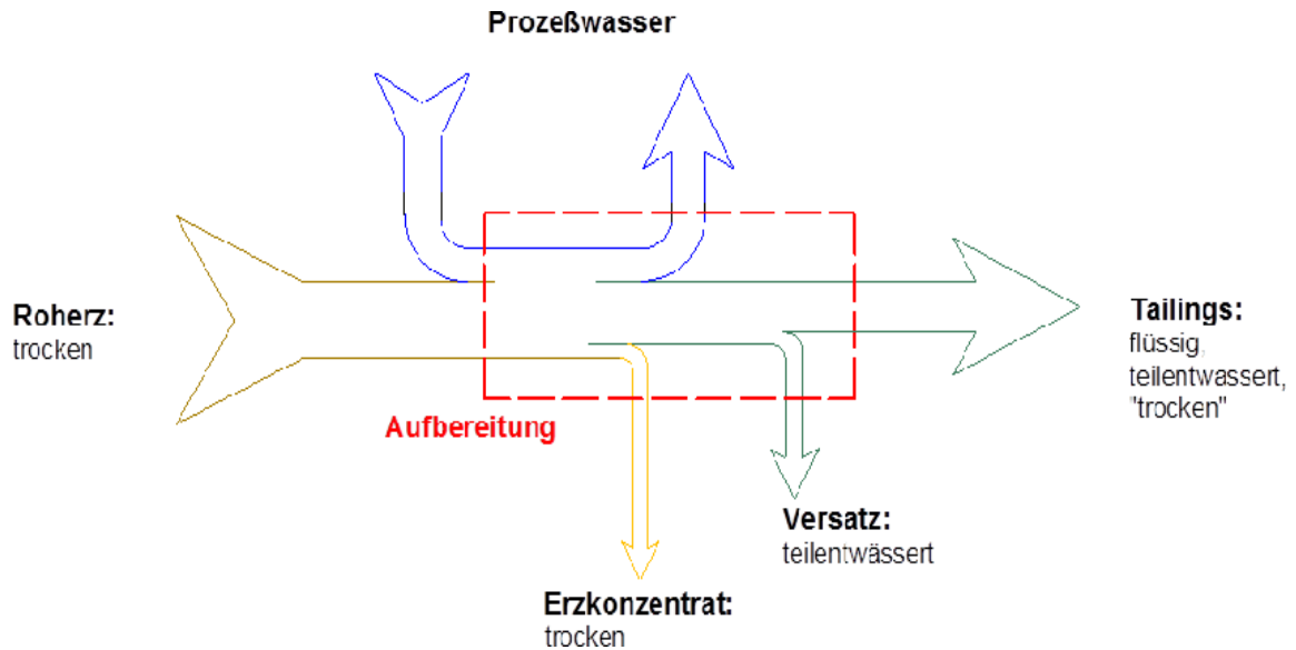
Abbildung 5: Stoffströme der Erzaufbereitung
