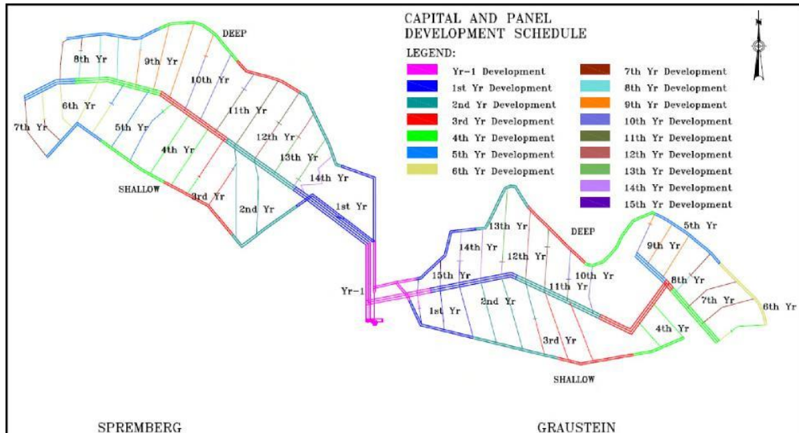
Abbildung 3: Jährliche Streckenauffahrung für Aus- und Vorrichtung
