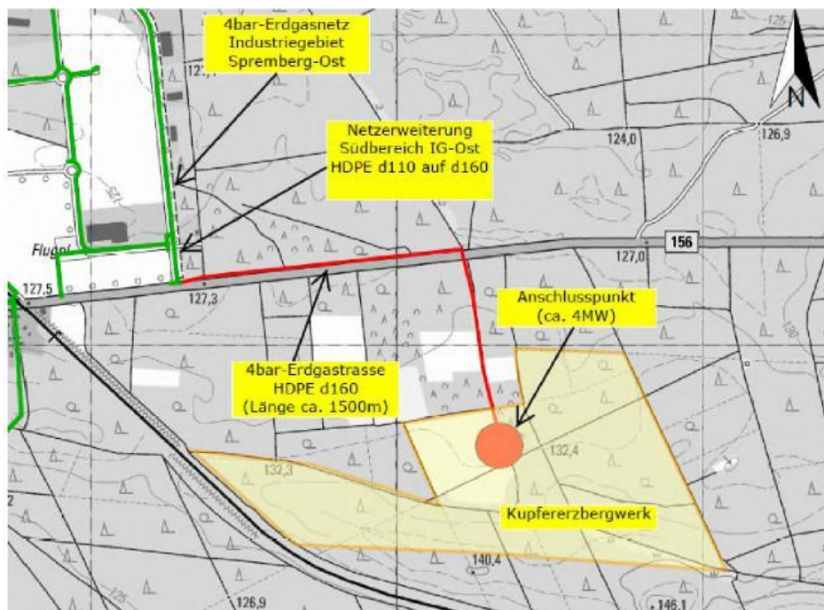
Abbildung 2: Anschluss an die Erdgasversorgung
