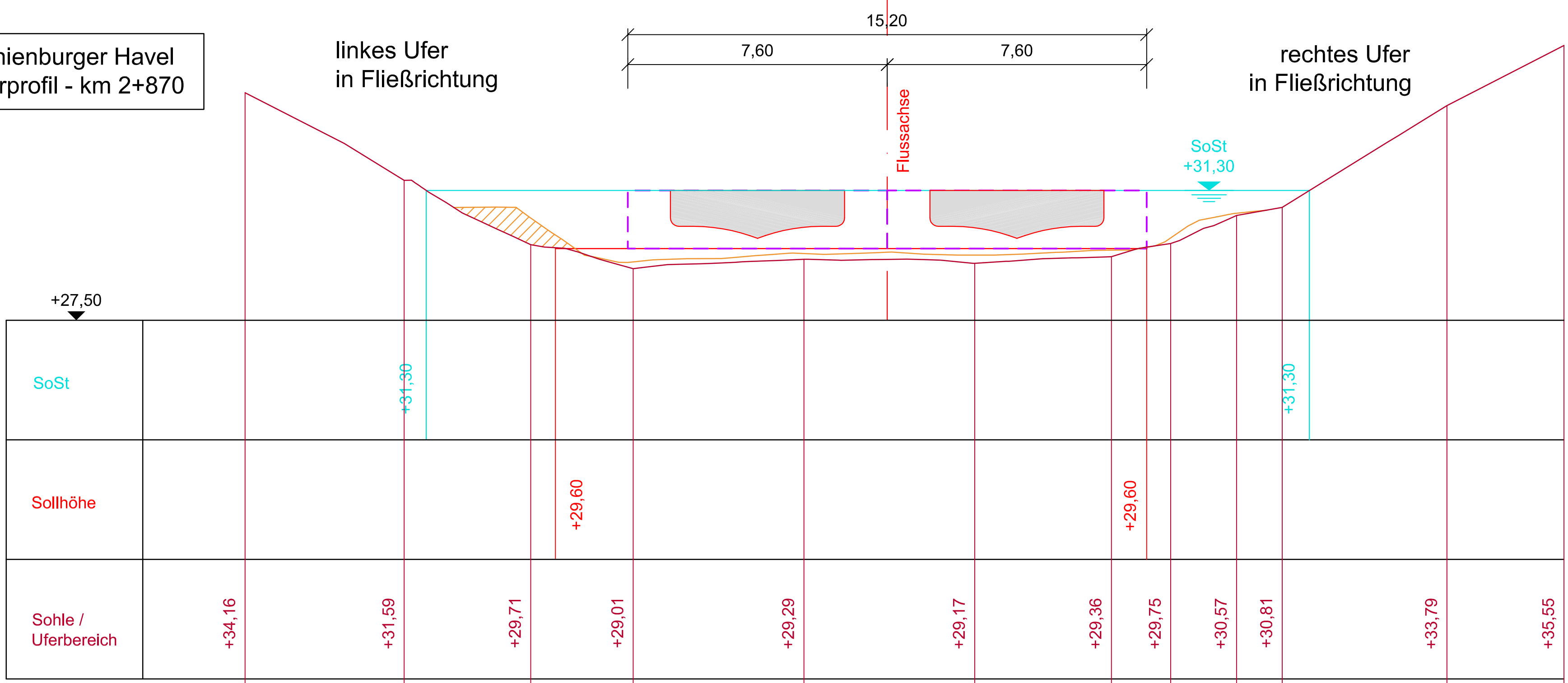
Oranienburger Havel Querprofil - km 2+720
