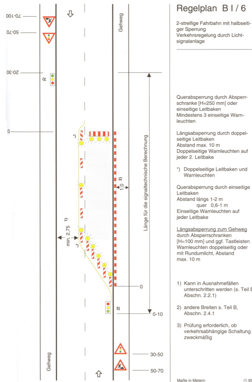
RSA 95 - Regelplan B I / 6
