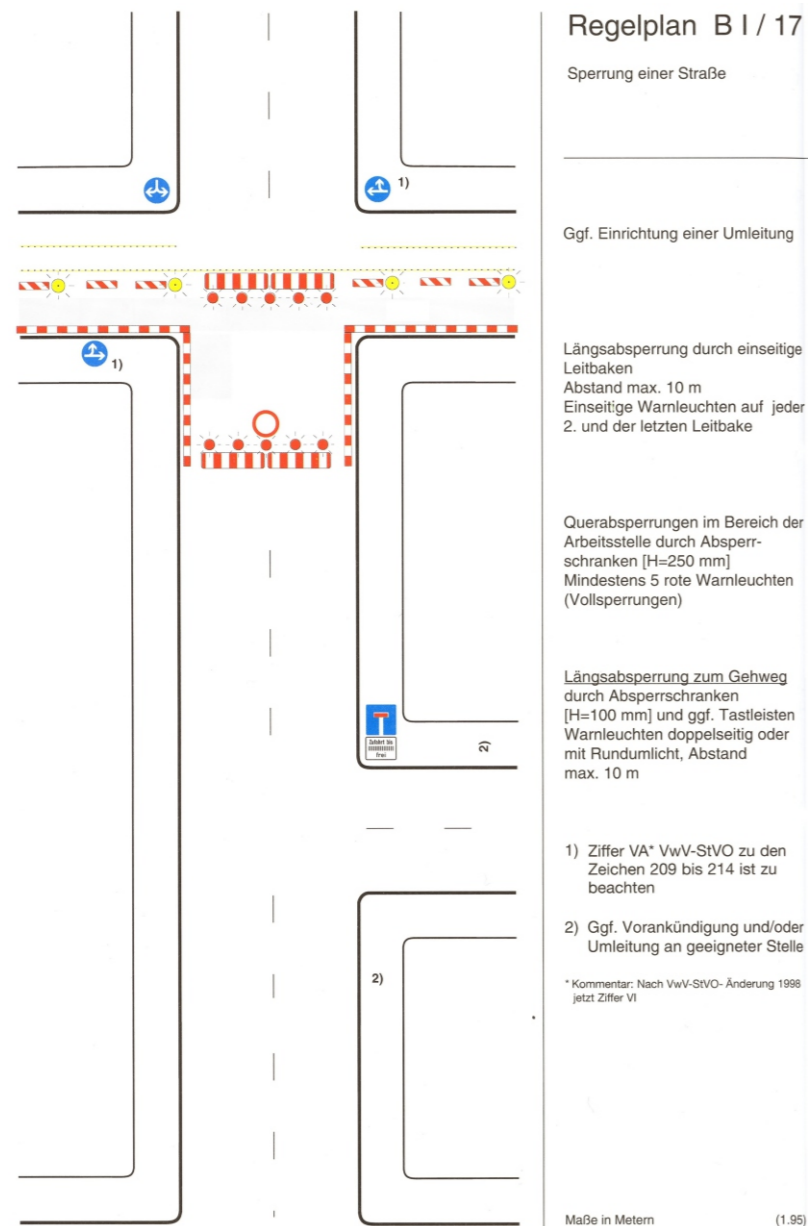
RSA 95 - Regelplan B I / 17
