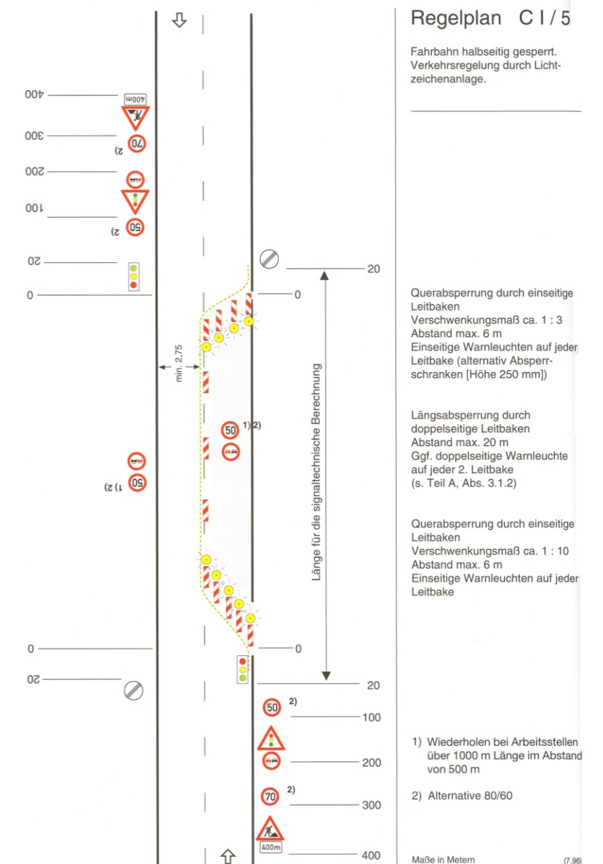
RSA 95 - Regelplan C I / 5
