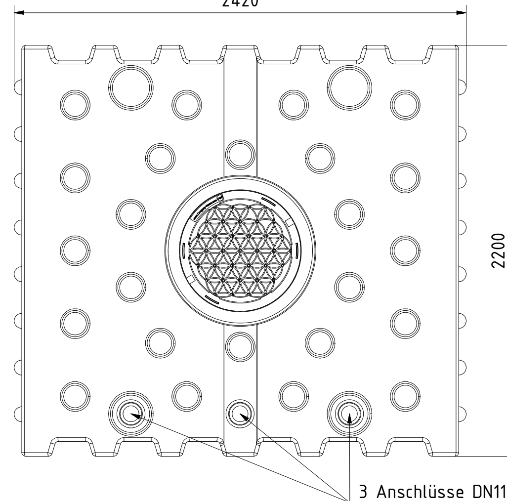
Draufsicht
