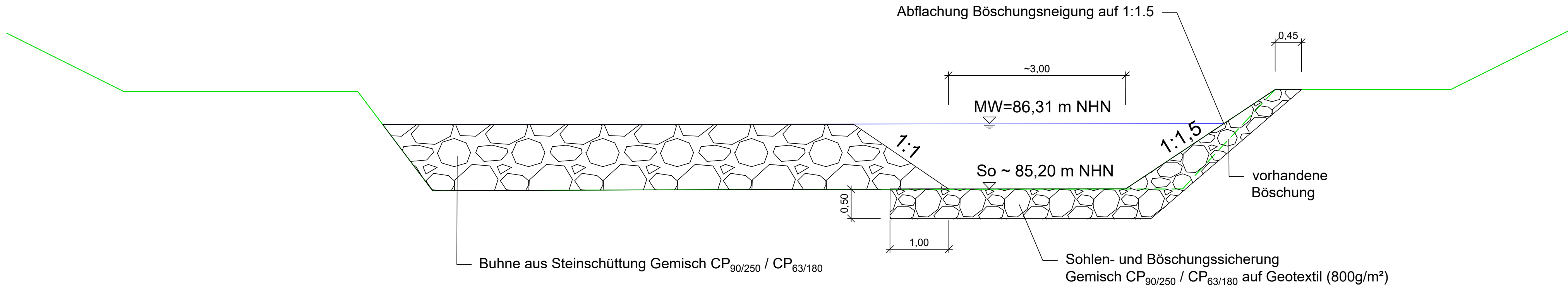
Schnitt Buhne M 1:50
