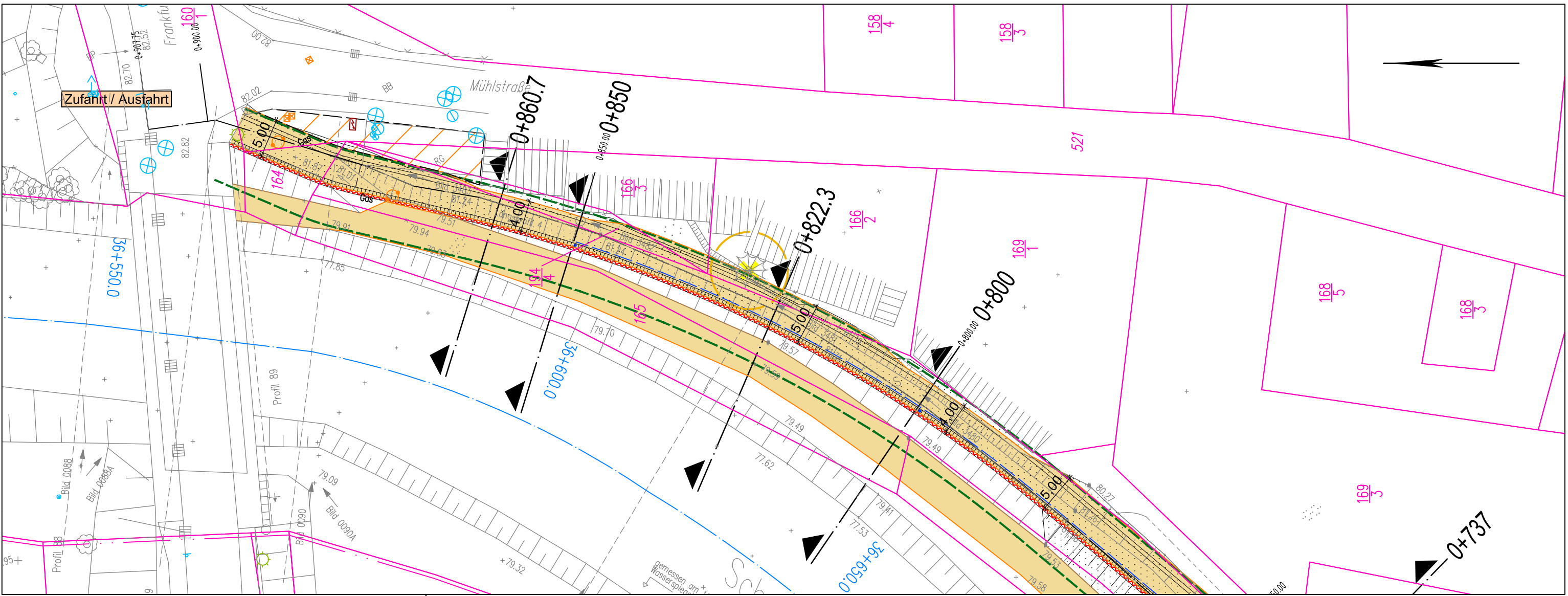
Lageplanausschnitt M 1 : 500
