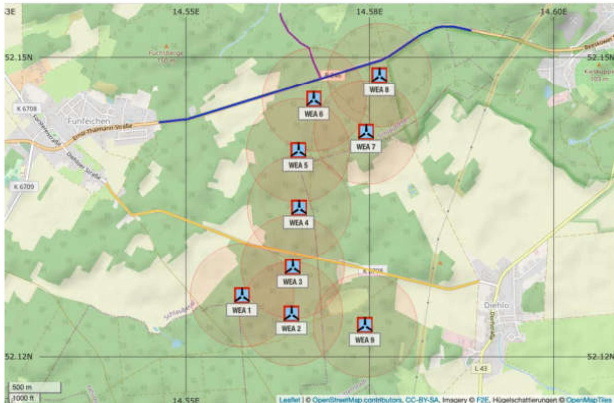
Abbildung 4.3.1: Potentielle Gefährdungsbereiche der WEA 1 - 9 und Schutzobjekte am Standort Schierenberg (Karte /1.4/).
