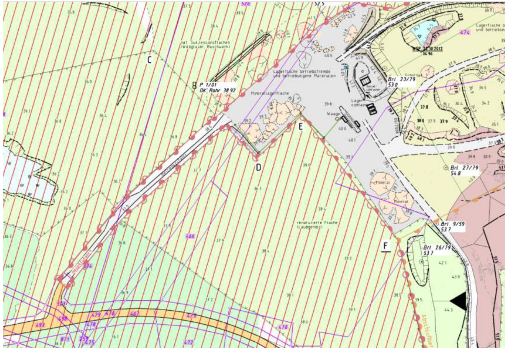
Abbildung 1: Ausschnitt aus dem Risswerk des Tagebaus Niederlehme mit Darstellung des Zufahrtbereichs und Bereich der Tagesanlage
