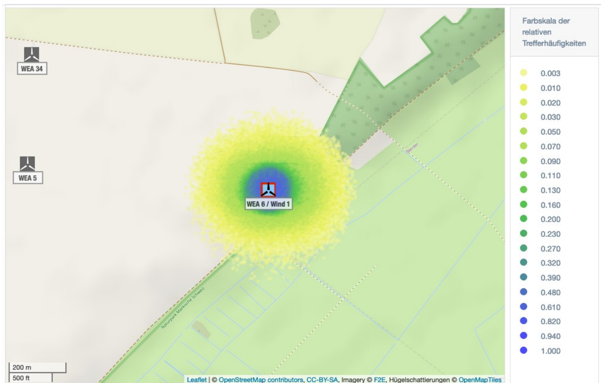
Abbildung B.1.1: Trefferhäufigkeiten von Eisstücken pro Rasterfläche (16m 2 ) und Jahr in der Umgebung der WEA 6 am Standort Zinndorf (Karte /1.4/).
