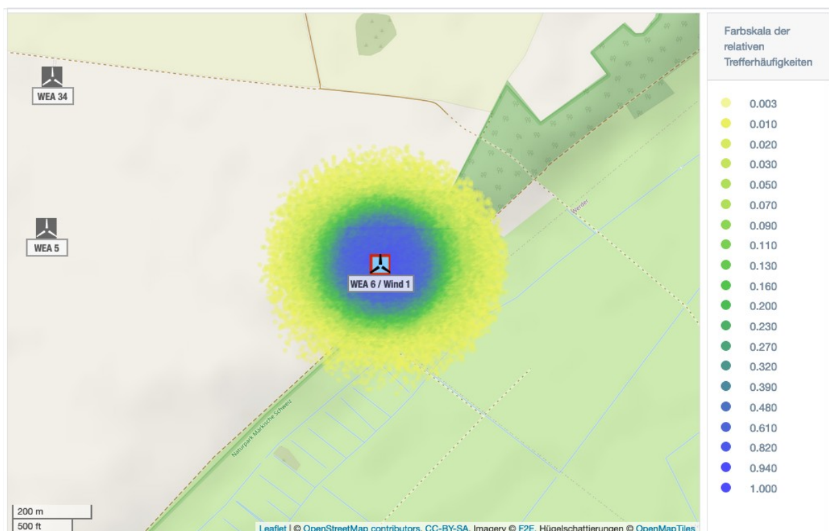
Abbildung A.1.1: Trefferhäufigkeiten von Eisstücken pro Rasterfläche (16m 2 ) und Jahr in der Umgebung der WEA 6 am Standort Zinndorf (Karte /1.4/).
